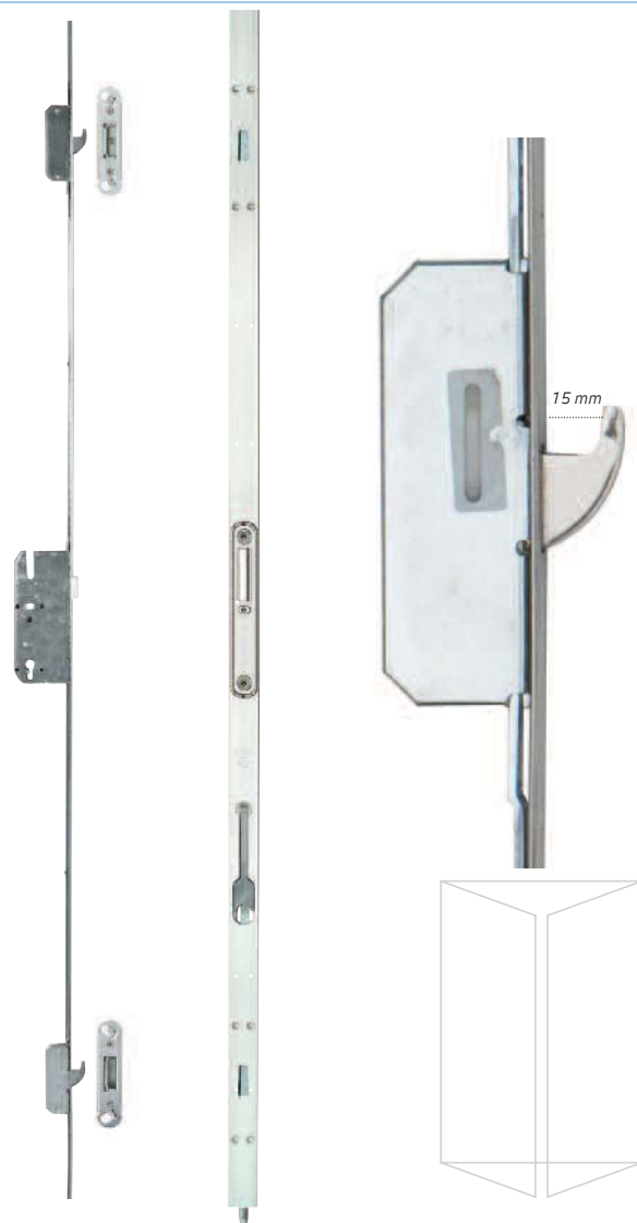
Stolpstel Inbraakwerend volgens NEN 5096 (klasse 3) Naar binnen/Naar buiten draaiend bereikbaar Espagnolet HaKo 3000/98MPD Stolpdeur
